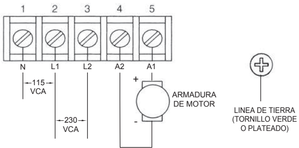
Figura 15. Conexiones para Controles con Gabinete
