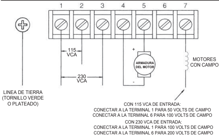
Figura 15. Conexiones para Controles con Gabinete
