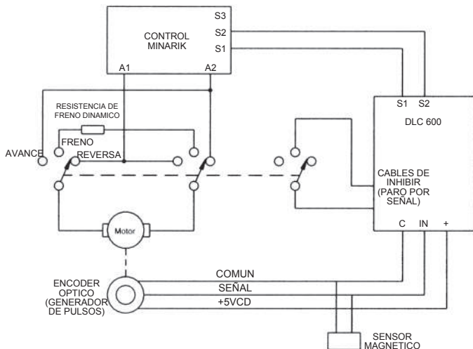
Figura 30. Reversa con un DLC600 (DIGI-LOK)
