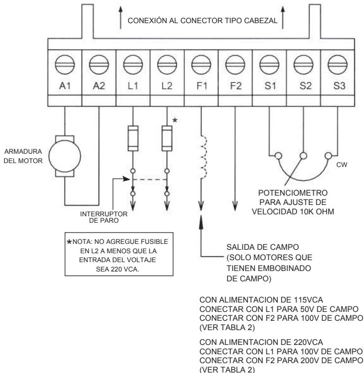
Figura 13. Conexiones para MM23201C-Q y MM23011C-Q
