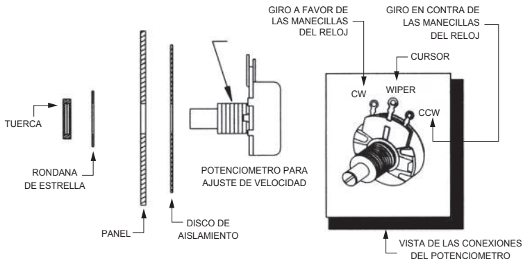
Figura 11. Potenciómetro para Ajuste de Velocidad
